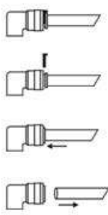
Poza 11. Deconectarea fittingului rapid de la tubul PE
