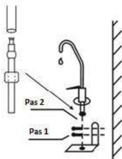
Poza 6. Robinetul pe peret
